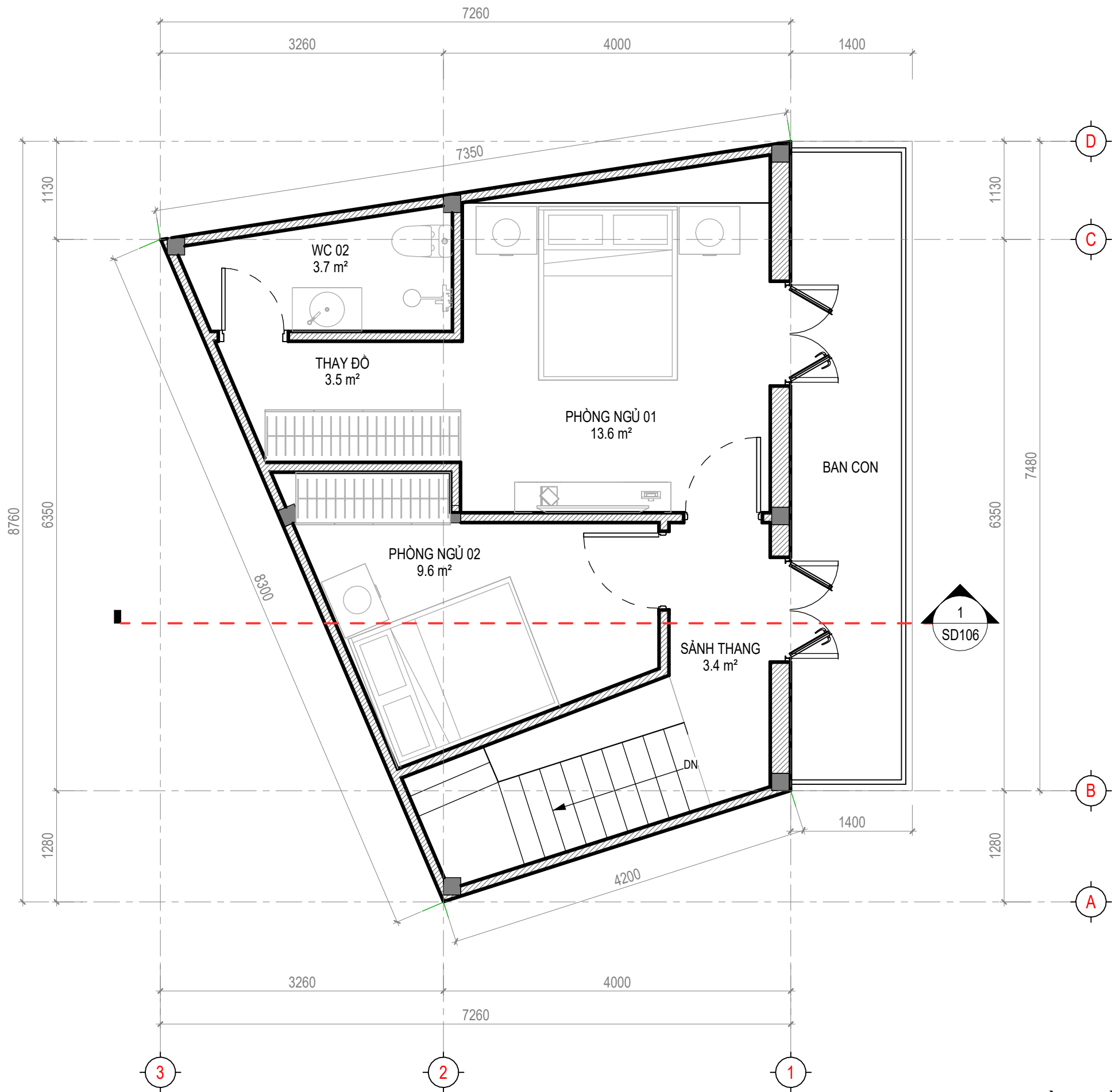
MẶT BẰNG TẦNG 2 TL 1 : 50
